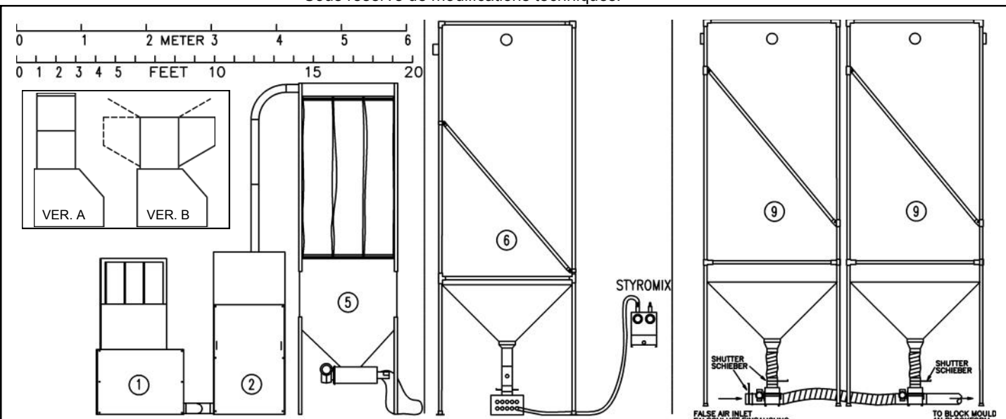
1. Prébroyeur et granulater combinés (avec boîtier d'insonorisation). 2. Unité de dépoussiérage. 5. Compacteur poussière pour PSE et PPE avec ramassage en sac. 6. Silo de stockage pour matière recyclée. STYROMIX: Mélange avant chaque machine de moulage. 9. STYROMETER Unité de dosage pour matière recyclée avant le moule à bloc ou pour mélange PPE avant le réservoir sous pression.
